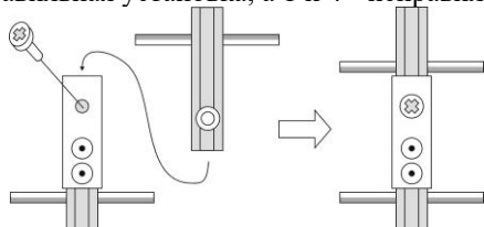
Рис. 2 Сборка антенны AX-1817Y
