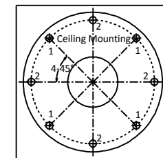
Рисунок 2-1 Шаблон крепления
